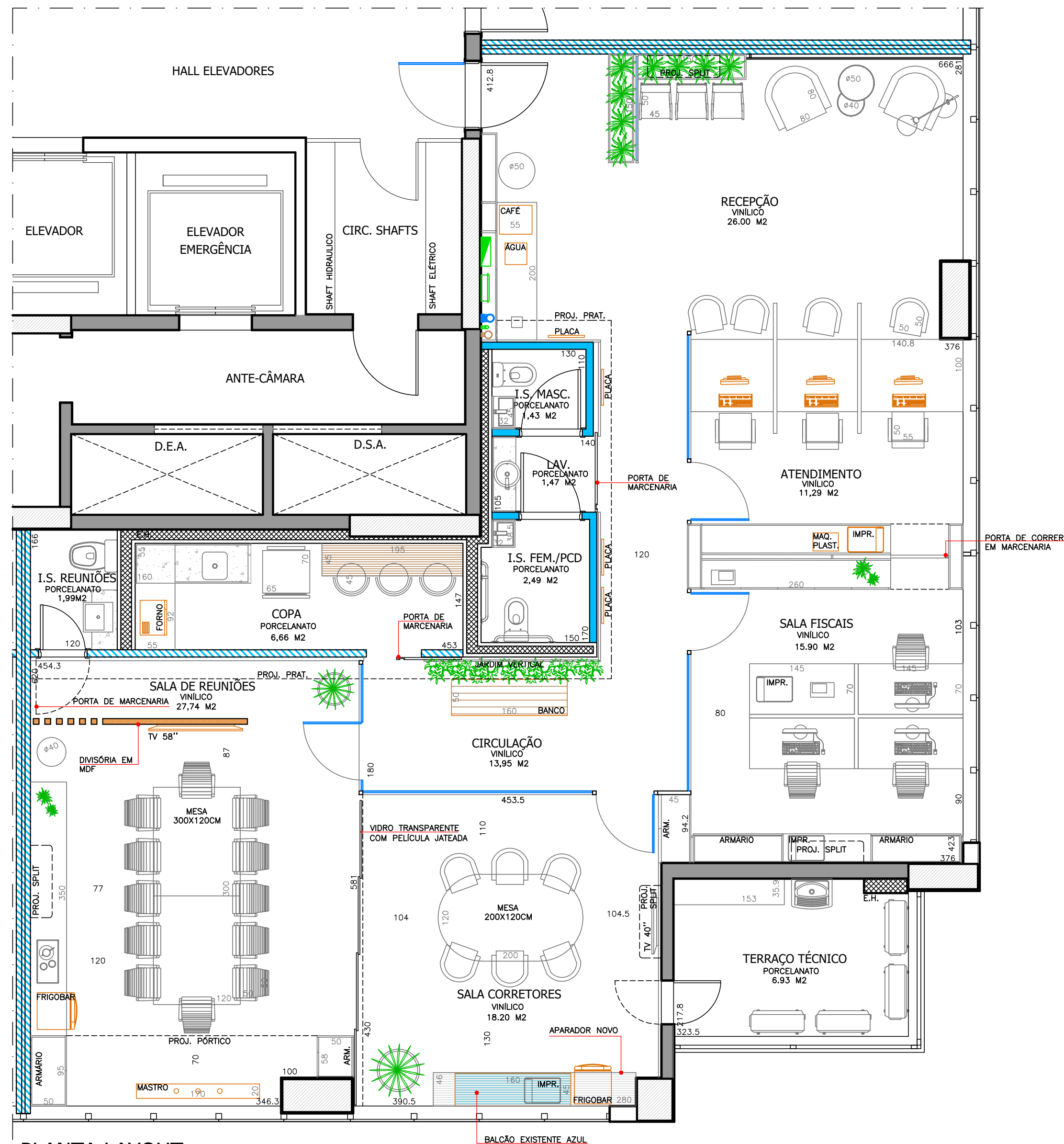
PLANTA LAYOUT ESCALA 1:50
