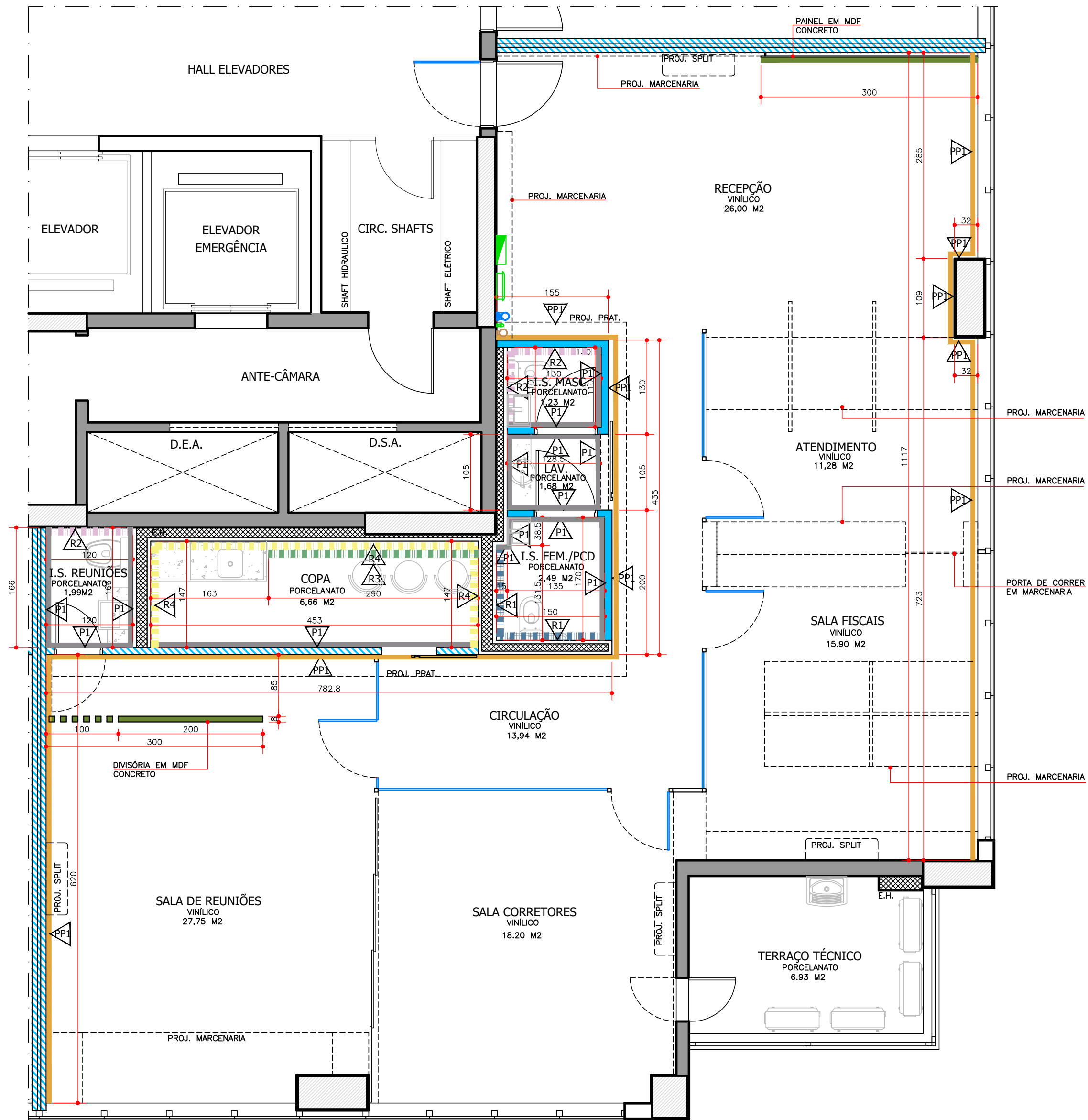
PLANTA LAYOUT ESCALA 1:50
