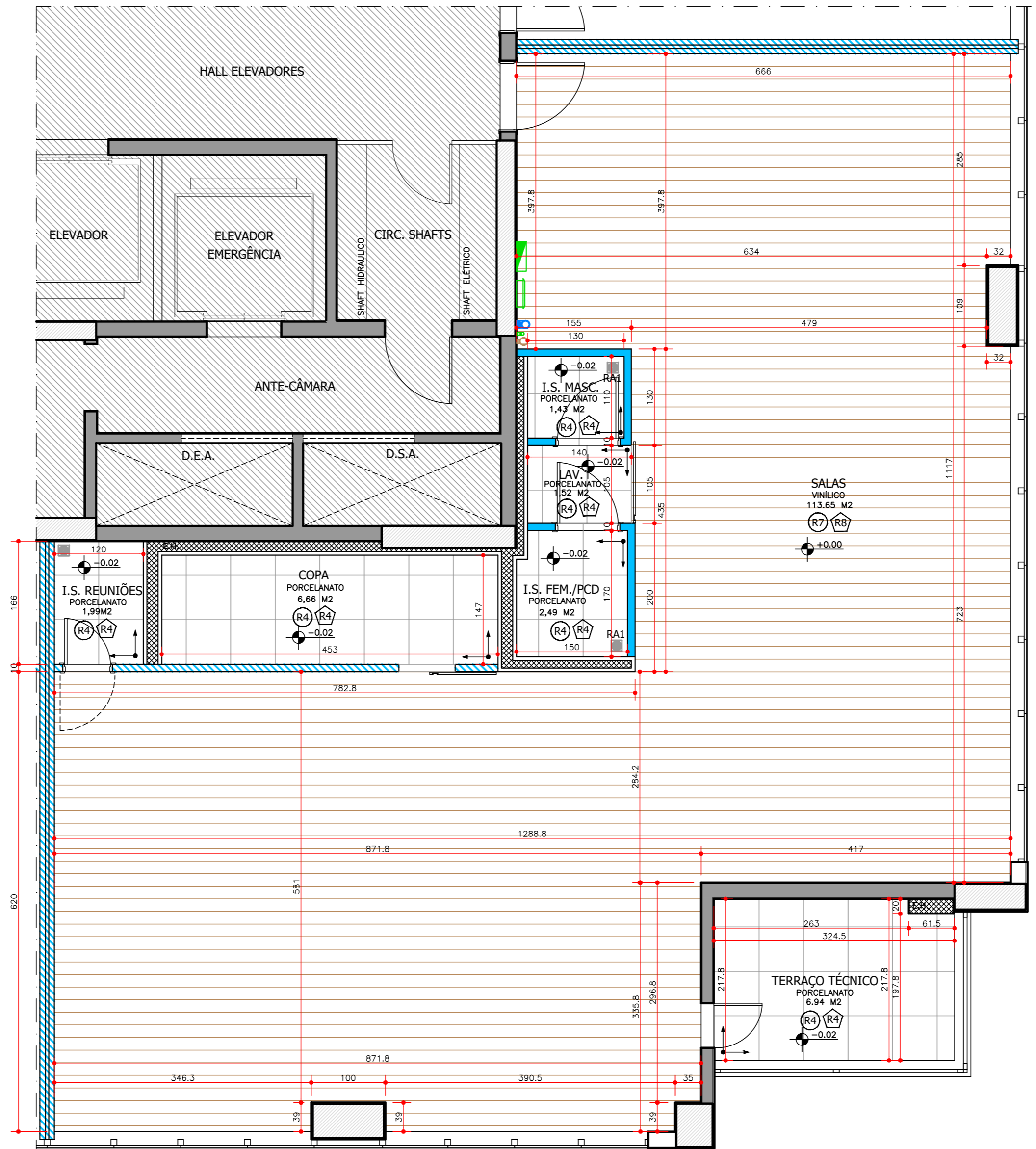
PLANTA DE PISO ESCALA 1:50
