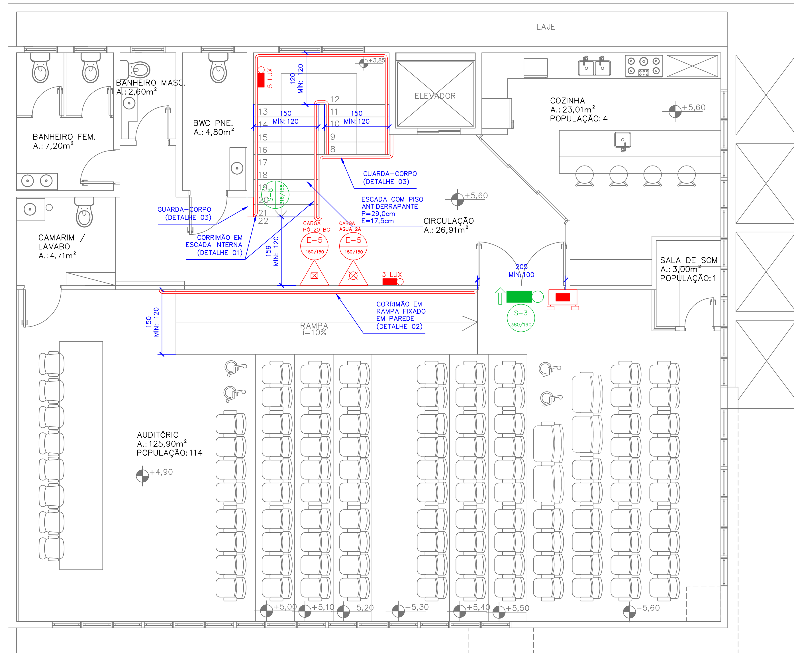
PLANTA BAIXA SUPERIOR ESCALA 1:50
