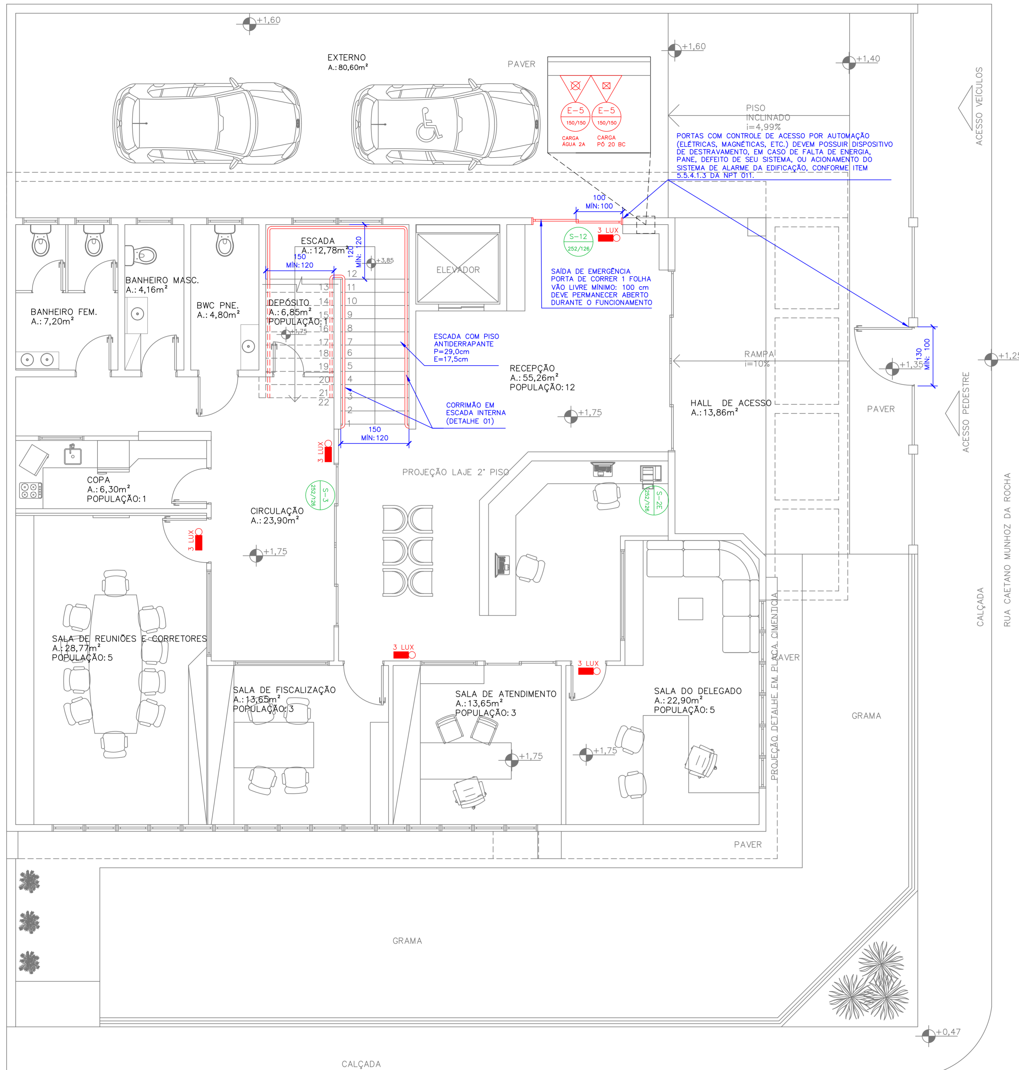
PLANTA BAIXA TERREO ESCALA 1:50
